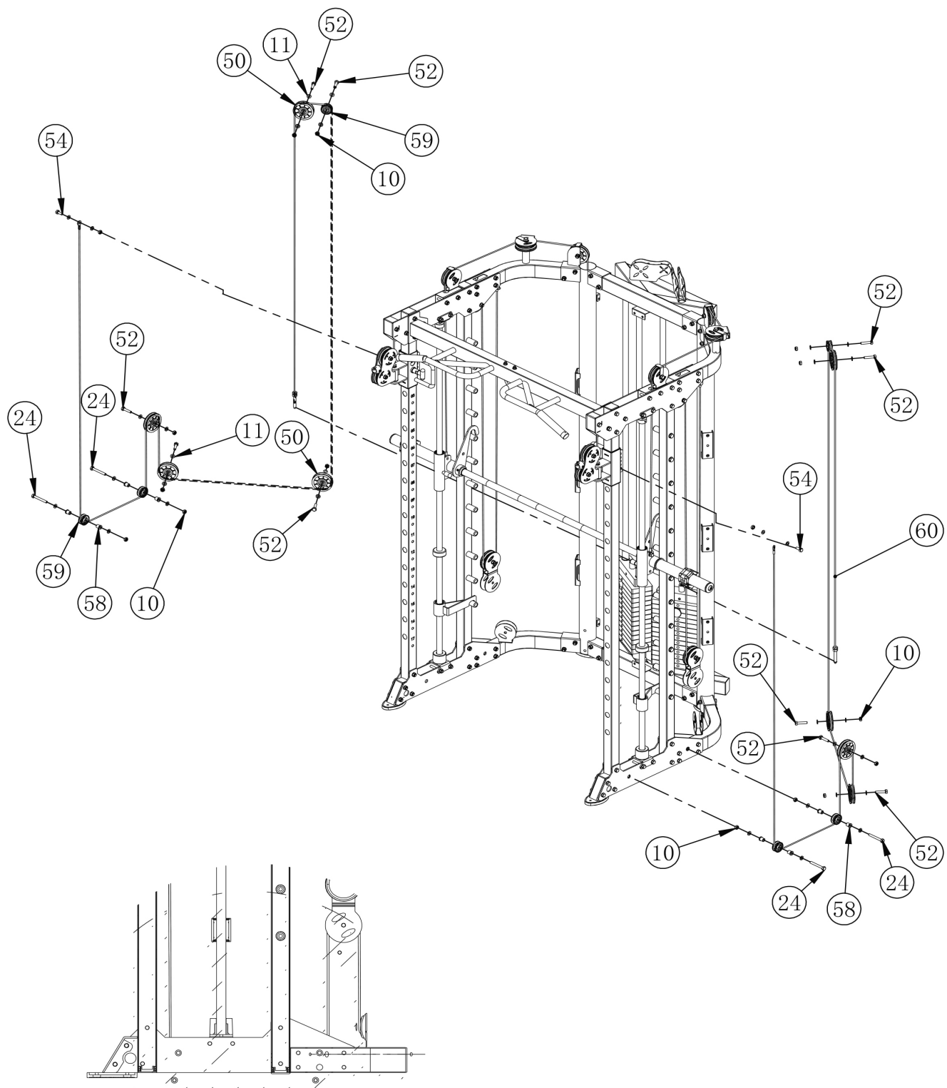
Kabelverlauf
