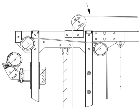
Kabelverlauf
